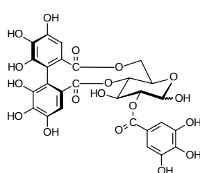
Hippomanin A ( 2 )
