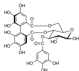
Gemin D ( 1 )
